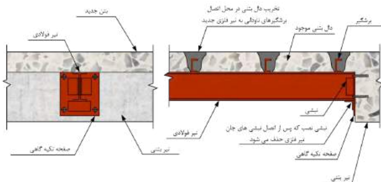
شکل ۱۴-۴۰- اجرای تیرک فولادی برای تقویت دال بتنی
