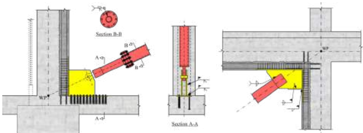
(الف) جزئیات اتصال ورق اتصال و مهاربندها به ناحیه اتصال
