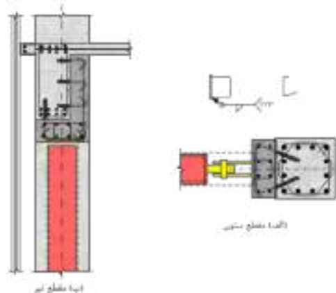
(پ) جزئیات تقویت المان‌های تیر و ستون به منظور نصب میراگر و مهاربندهای مربوطه (در صورت لزوم)
