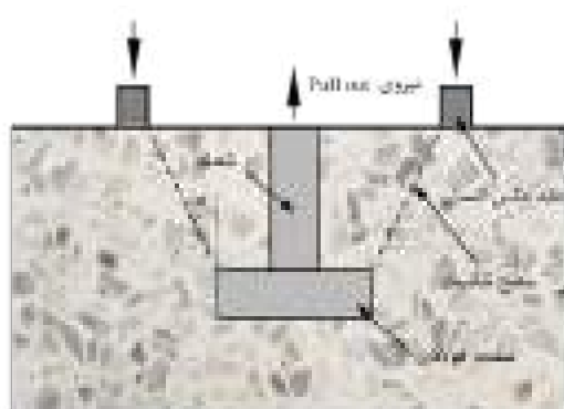
شکل ۱۴-۱- آزمایش بیرون‌کشیدگی (Pull Out) - روش اول
