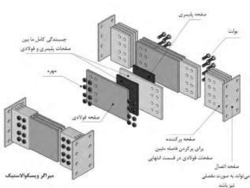
شکل ۱۴-۱۳۱- جزئیات یک نمونه میراگر ویسکوالاستیک
