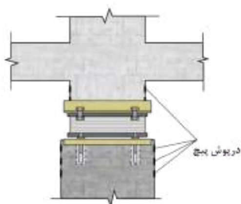
(۴) تزریق گروت انبساطی با جک تخت در فضای بین جداساز و ستون، باربرداری از جک‌های هیدرولیکی و انتقال بار از پایه‌های موقت به جداساز و نهایتاً برچیدن پایه‌های موقت و پوشاندن کوپلرها با درپوش
