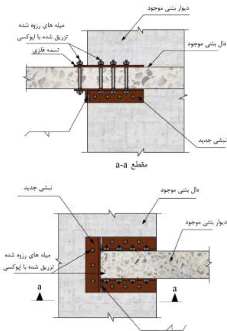
شکل ۱۴-۲۵- تقویت دیوار بتنی در محل اتصال به دال
