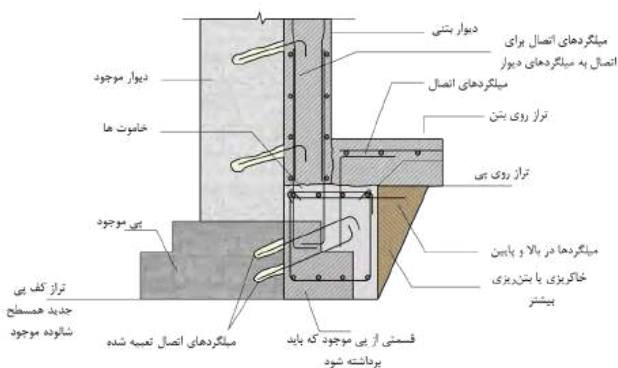
شکل ۱۴-۱۱۵- اجرای پی نواری بتنی جدید در کنار پی نواری موجود
