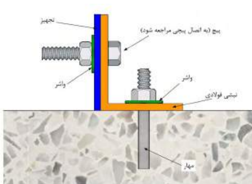
شکل ۱۴-۱۹۸- اتصال مهار با قطر بیشتر از ۱۰ mm به تجهیزات
