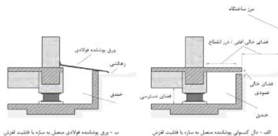
شکل ۱۴-۱۶۱- روش‌های مختلف پوشاندن درز حرکتی
