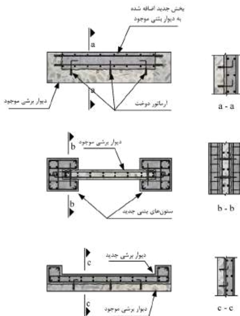
شکل ۱۴-۳۶- تقویت دیوارهای برشی موجود
