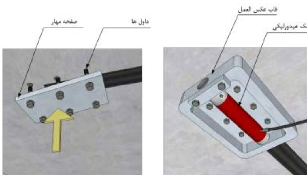
شکل ۱۴-۶۲- نصب جک جهت اعمال پیش تنیدگی
