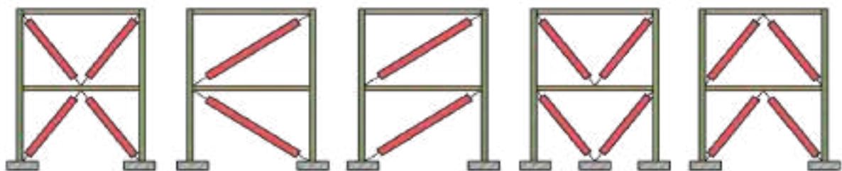
الف- مهاربندی هشتی ب- مهاربندی هفتی ب- مهاربندی قطری ت- مهاربندی قطری ث- مهاربندی ضربدری (زیگزاگ) چند طبقه
