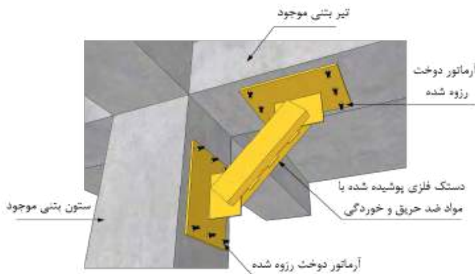
شکل ۱۴-۲۸- استفاده از دستک‌های فلزی در تقویت اتصالات تیر به ستون بتنی مسلح
