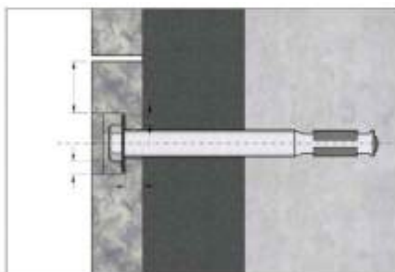
شکل ۱۴-۱۷۴- جزئیات مهار سطحی به وسیله اتصال مکانیکی در روی سنگ
