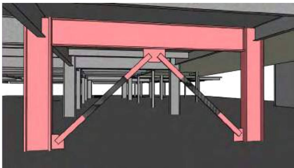
شکل ۱۴-۱۰۲- تقویت مهاربند با FRP
