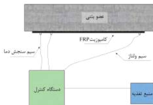
شکل ۱۴-۴۸- ایجاد گرمایش جهت عمل آوری سریع با استفاده از ظرفیت رسانایی کامپوزیت‌های CFRP
