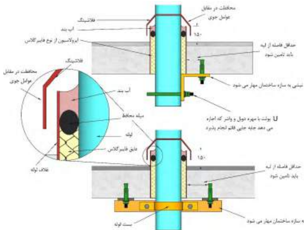
شکل ۱۴-۱۹۵- جزئیات نگهدارنده لوله قائم در بام
