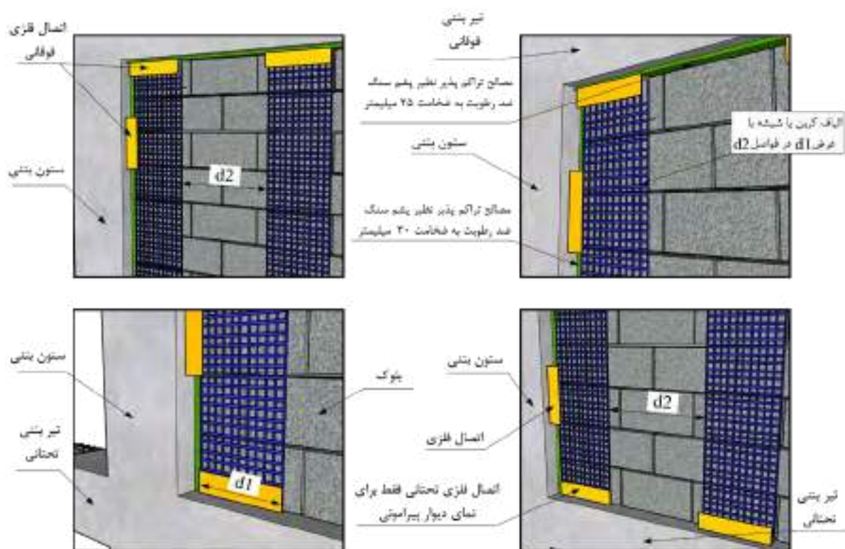
شکل ۱۴-۱۸۲- جزئیات بهسازی لرزه‌ای دیوارها با شبکه ایاف
