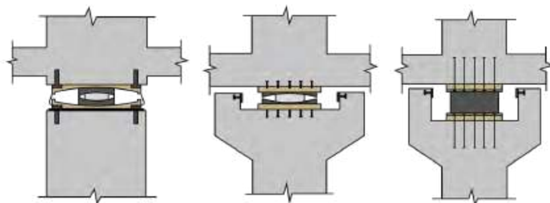
الف- جداساز لاستیکی با هسته سربی ب- جداساز اصطكاكي تك پاندولی پ- جداساز اصطكاكي سه پاندولی شكل ۱۴-۱۵۳- جزئیات نصب ایمن انواع مختلف جداسازها در بالای ستون با پایه‌های اطمینان یا رینگ محافظ پیرامونی
