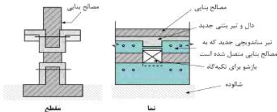
الف - تیرهای ساندویچی جدید ساخته شده و یک پازشو برای نصب جداساز ایجاد می گردد
