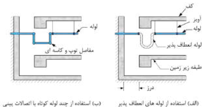
شکل ۱۴-۱۷۰- جزئیات اجرای لوله‌کشی‌ها در ساختمان جداسازی شده
