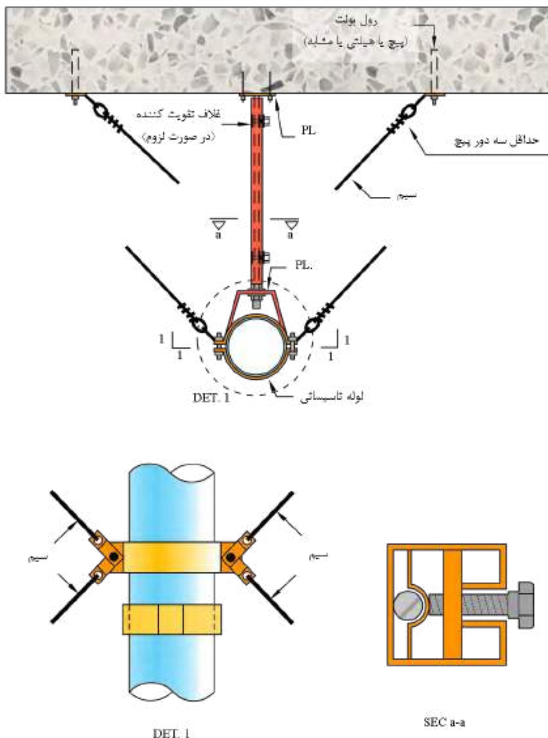
شکل ۱۴-۱۹۲- جزئیات مهار لوله‌های تأسیساتی
