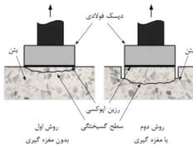
شکل ۱۴-۳- آزمایش کشش سطحی (Pull Off)
