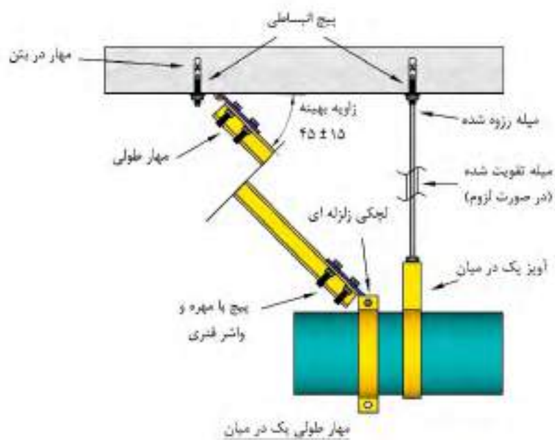
شکل ۱۴-۱۹۳- جزئیات مهر تک لوله
