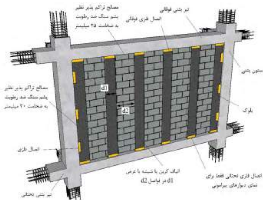
شکل ۱۴-۱۸۱- بهسازی لرزه‌ای دیوارها با استفاده از نوارهای شبکه ایاف
