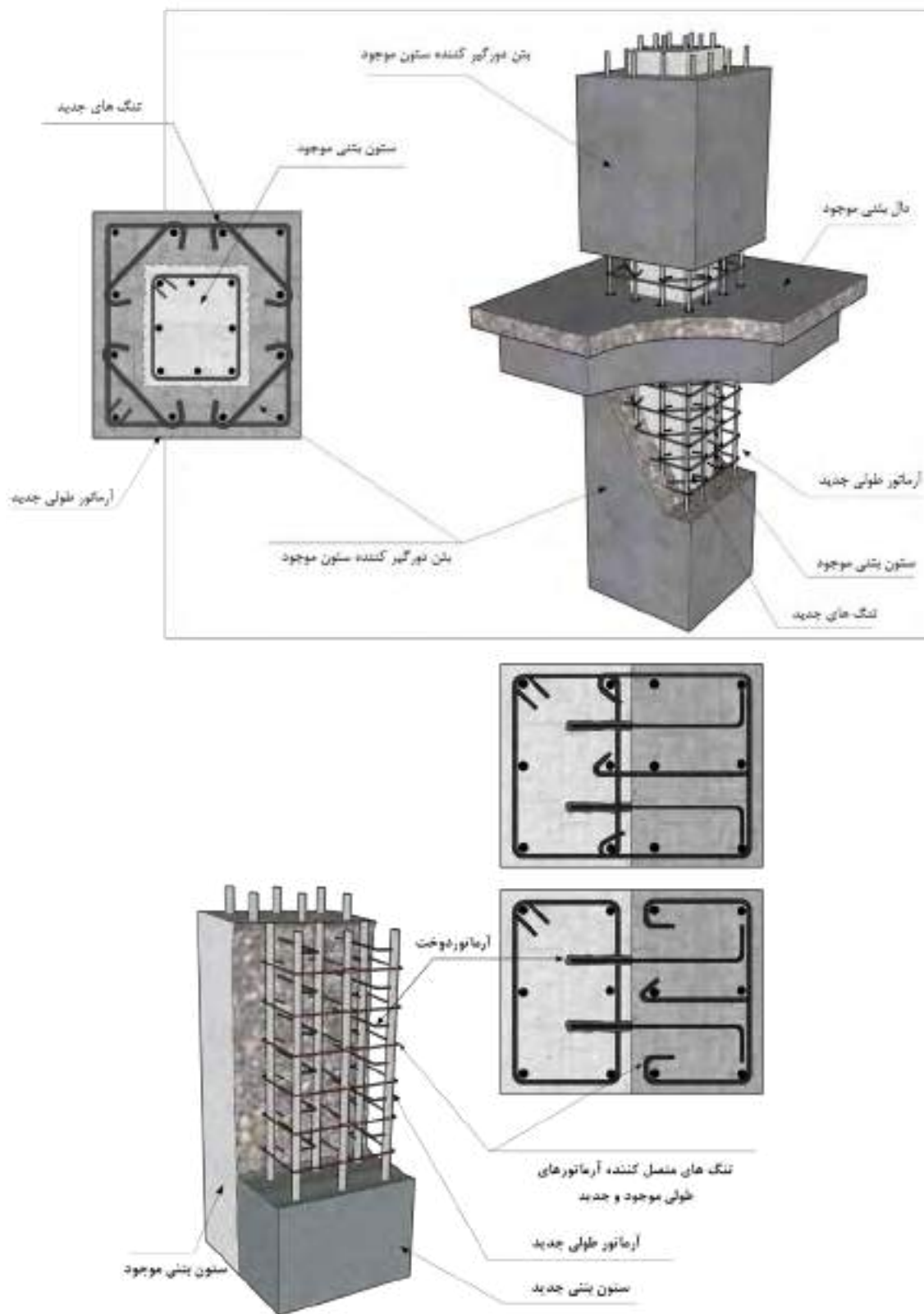
شکل ۱۴-۱۴- تقویت ستون بتنی با استفاده از ژاکت بتنی
