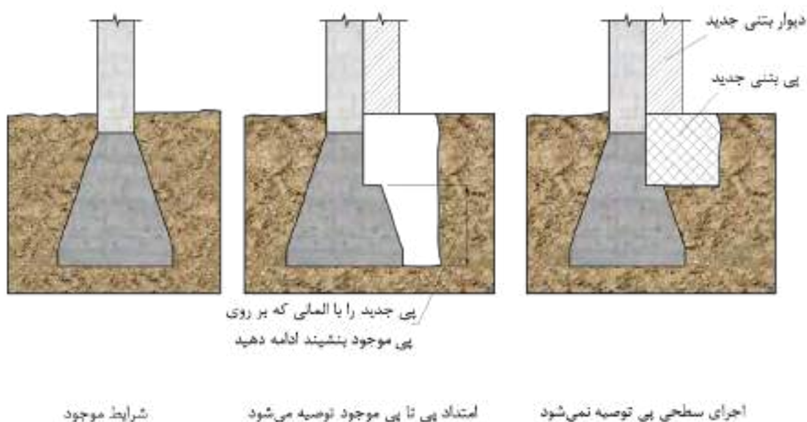
شکل ۱۴-۱۱۷- اجرای پی سطحی جدید در عمق کمتر از پی سطحی موجود
