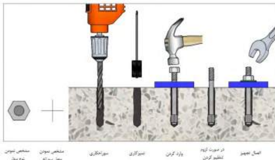
شکل ۱۴-۱۹۶- مراحل نصب مهارهای غیر چسبنده
