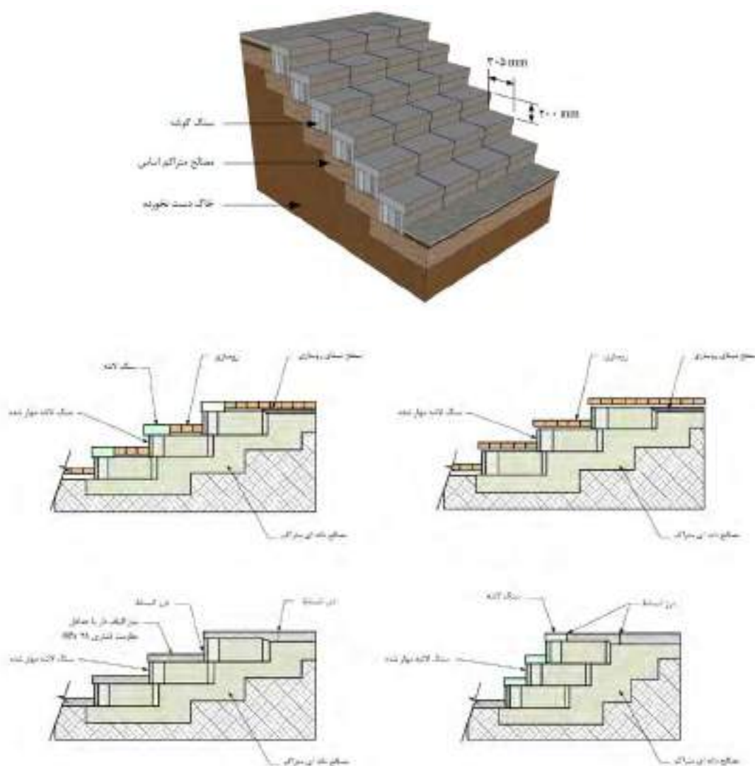
شکل ۱۳-۱۷- انواع پله
