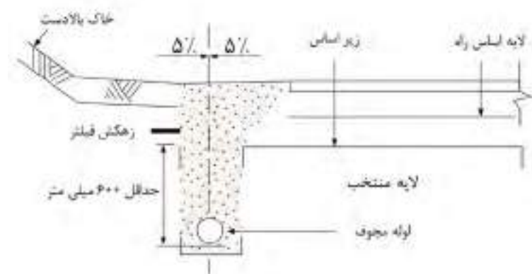
شکل ۱۳-۲۲- نمونه شماتیک سیستم زهکشی سطحی ترکیبی (فرانسوی)
