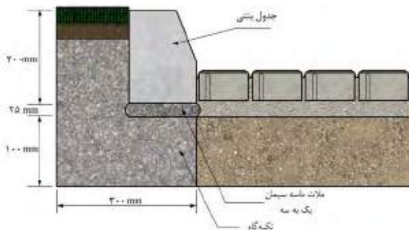
شکل ۱۳-۹- تکیه گاه در معابر و توقفگاه ها
