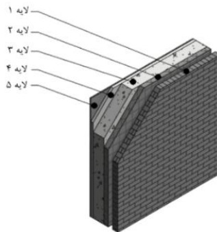
شکل ۱۹-۵: نحوه محاسبه مقاومت حرارتی پوسته خارجی غیرنورگذر چند لایه
