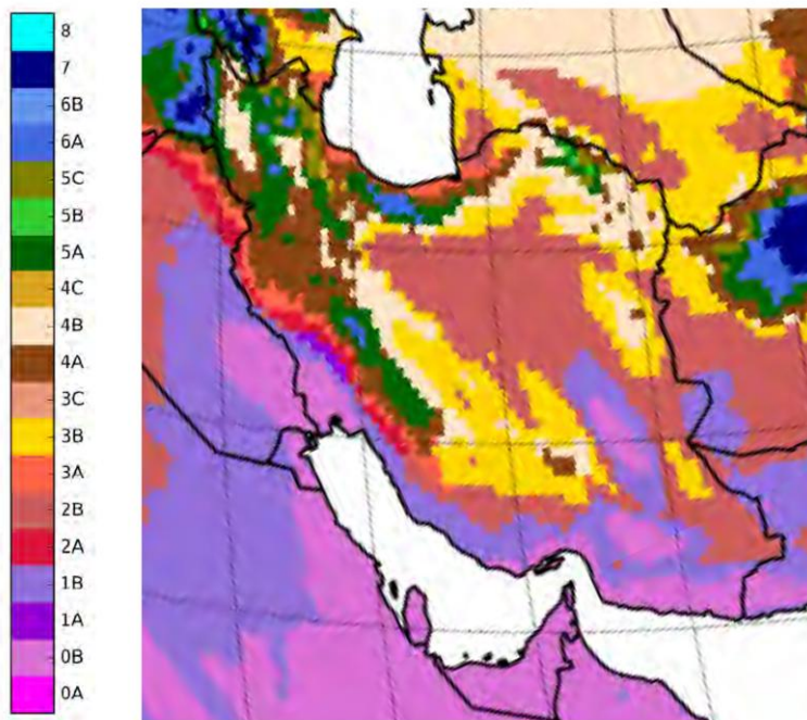
شکل ۱۹-۳-۲: دسته‌بندی اقلیمی در پهنه جغرافیایی ایران
