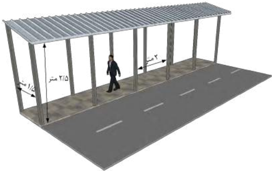
شکل ۲-۱- راهرو سرپوشیده موقت
