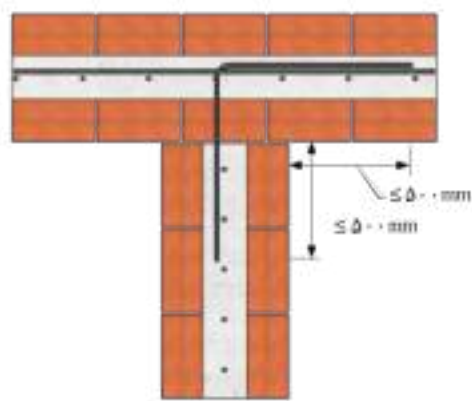
شکل ۸-۱۴- ضوابط مهار میلگردها در محل تقاطع دیوار بنایی مسلح
