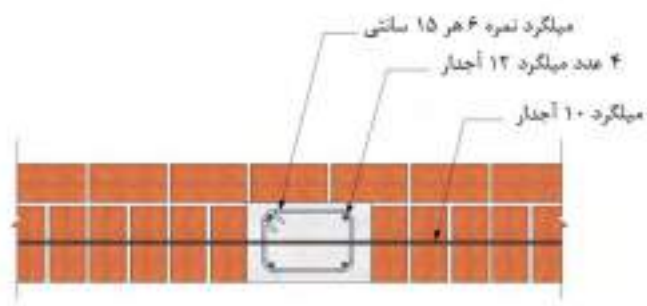
الف- پلان عبور میل گرد طولی از دیوارهای در یک امتداد
