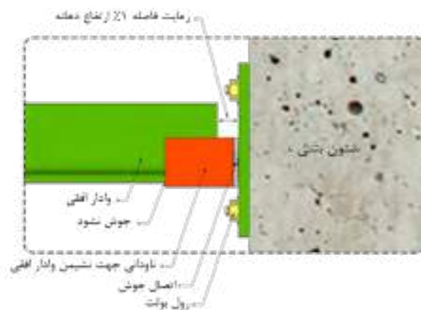
شکل ۸-۳۸- جزئیات اجرایی اتصال تیرک و وادی در دیوار با ارتفاع بیش از ۳/۵ متر
