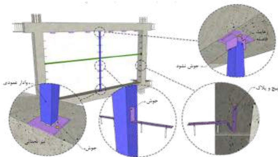
شکل ۸-۳۷- دیوارهای بلوکی با ارتفاع بیش از ۳/۵ متر دارای تیرک و وادی
