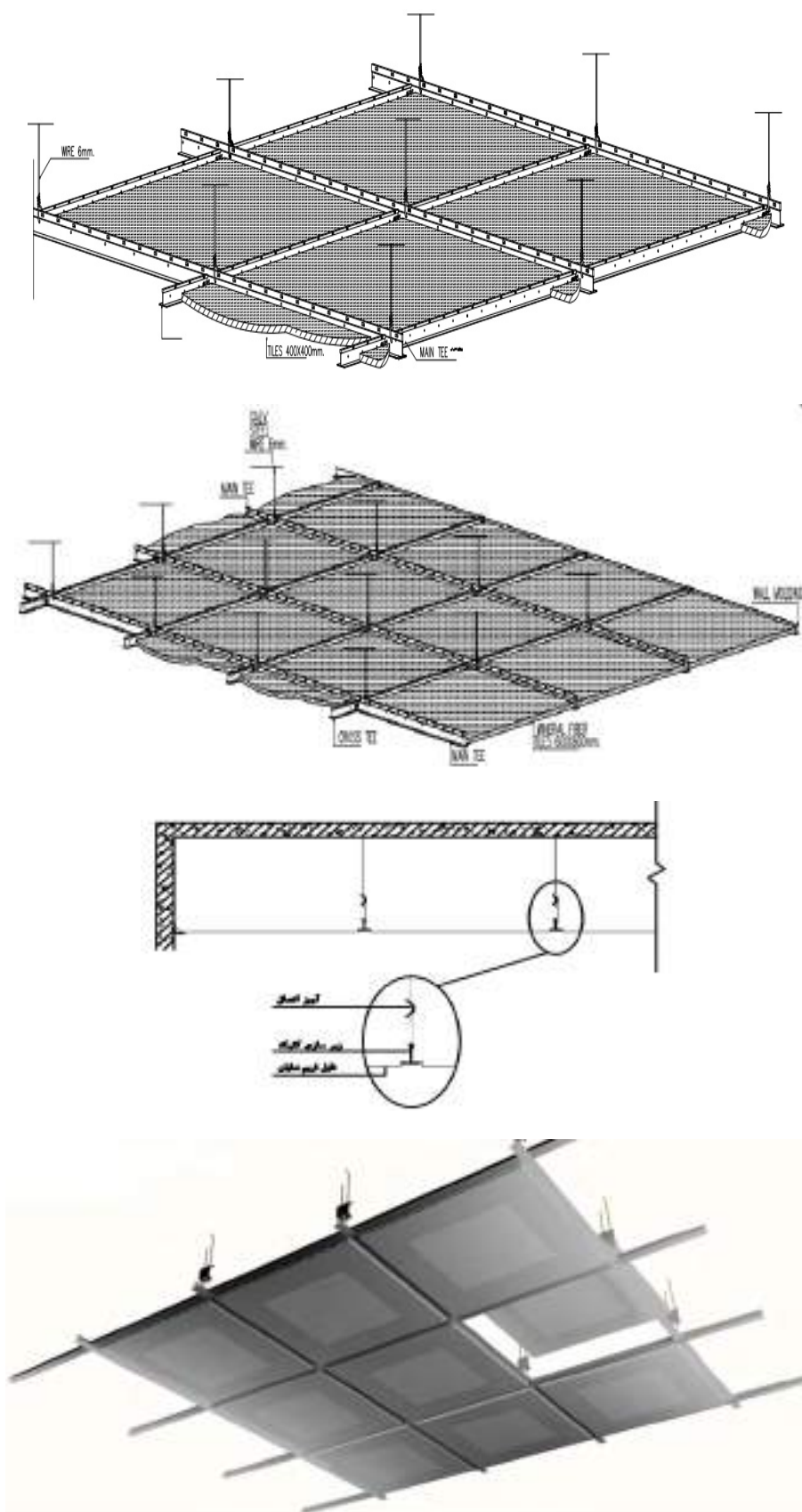
شکل ۸-۷۶- سقف کاذب از نوع تایل آلومینیومی با زیر سازی کلیک نمایان و نمونه اجرا شده آن
