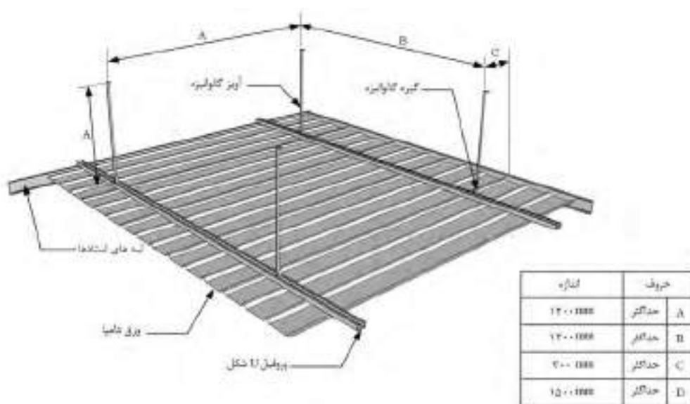
شکل ۸-۷۸- سقف کاذب دامپا
