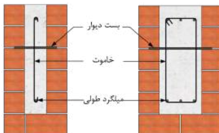
شکل ۸-۱۵- نمونه‌هایی از اجرای تیرهای بنایی مسلح (مقاطع)
