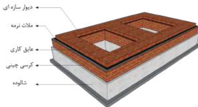
شکل ۸-۶- موقعیت کرسی چینی در اجزای ساختمان
