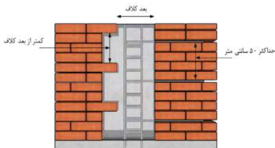
شکل ۸-۸- آرماتورهای جایگزین هشت‌گیر (وجه راست شکل) و فاصله بین واحدهای بنایی هشت‌گیر (وجه چپ شکل)
