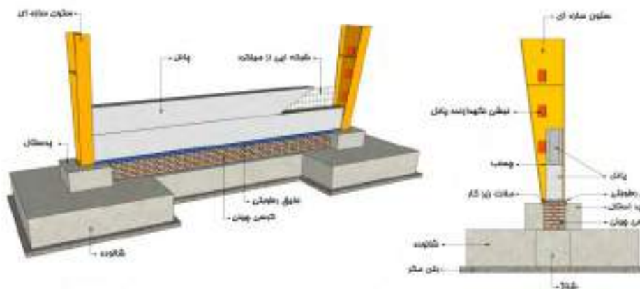
ب- نمونه دیوار پانلی افقی
