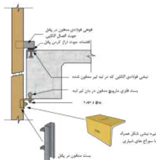
ب- نمونه اجرای اتصال لوبیایی به تیر در پانل بتنی پیش‌ساخته
