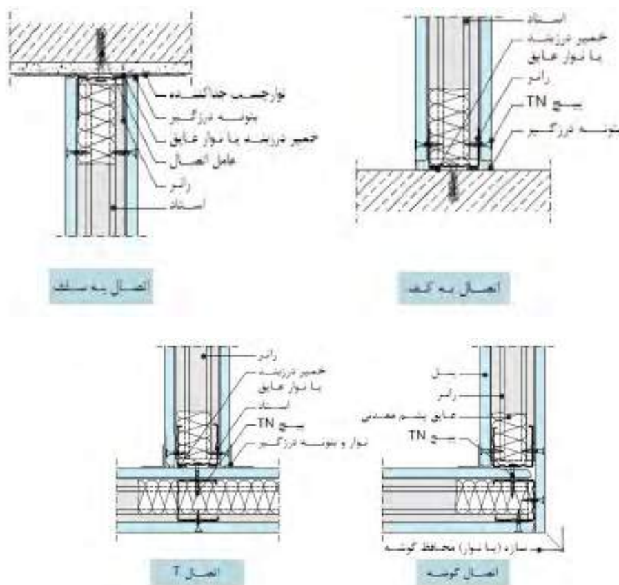
شکل ۸-۶۷- جزئیات نصب دیوار
