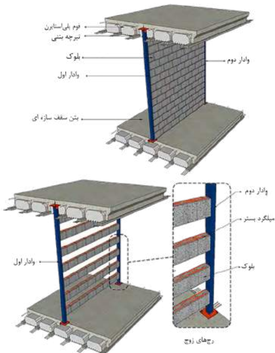
ب- عدم اتصال به سقف و اجرای المان مسلح کننده در رچ آخر دیوار
