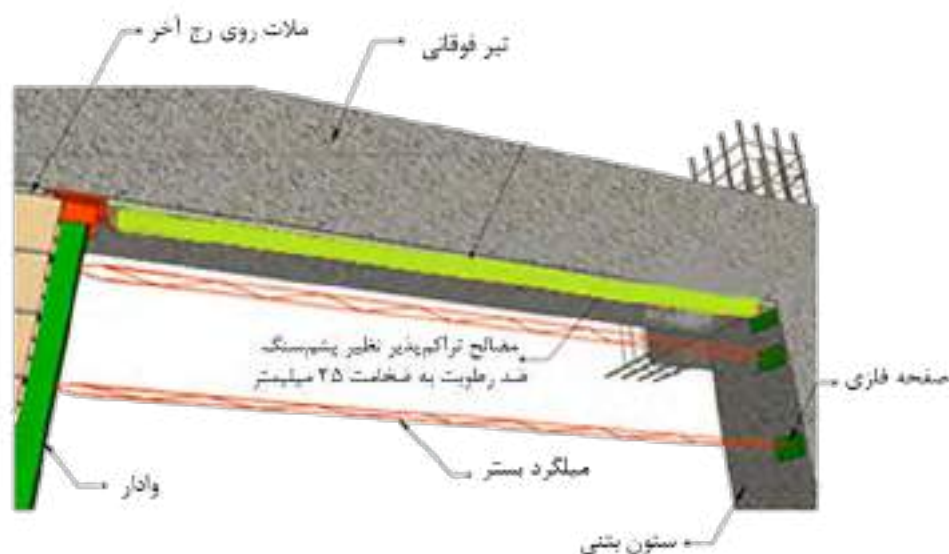
شکل ۸-۴۲- مهار دیوار به صورت یک طرفه با استفاده از قطعه مسلح کننده در بالاترین ردیف بلوک مصالح بنایی (اتصال وادار به سقف باید صورت کشویی باشد)
