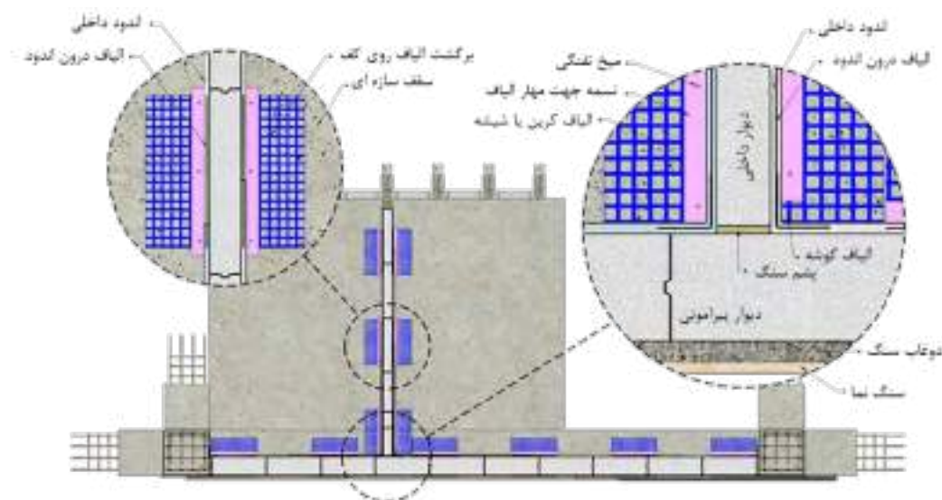
شکل ۸-۴۸- نحوه اجرا و تسلیح دیوارهای متقاطعات با استفاده از مش الایف
