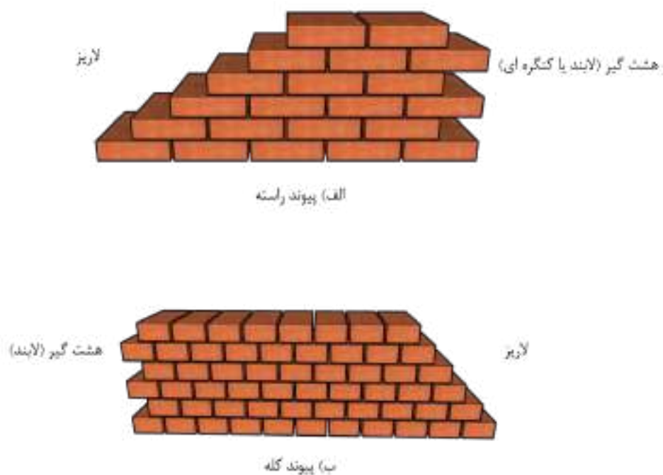
شکل ۸-۷- اتصال هشت‌گیر (لابند یا کنگره‌ای) و لاریز
