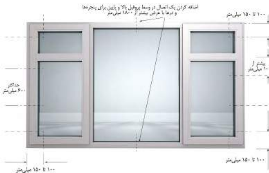
شکل ۱۲-۳۸- محل اتصالات پنجره‌ها و درهای آلومینیومی
