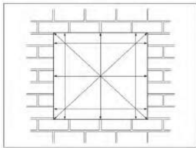
شکل ۱۲-۲۶- نحوه اندازه‌گیری ابعاد گشودگی
