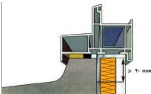
۴۵-۱۲- فاصله حداقل ۴۰ میلی‌متر نقاط اتصال نبشی از لبه بالایی (فوقانی) در مجاورت زیرپنجره یا پاخور در اجراشده در جا شکل
