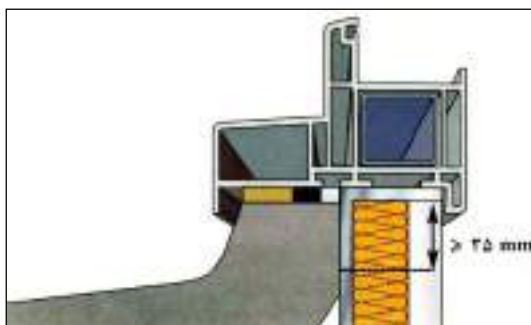
شکل ۱۲-۴۶- فاصله حداقل ۳۵ میلی‌متر نقاط اتصال نبشی از لبه بالایی (فوقانی) در مجاورت زیرپنجره پیش‌ساخته
