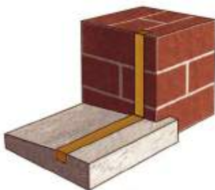
شکل ۱۲-۴۰- کاربرد پیش‌قاب چوبی در روش نصب توکار
