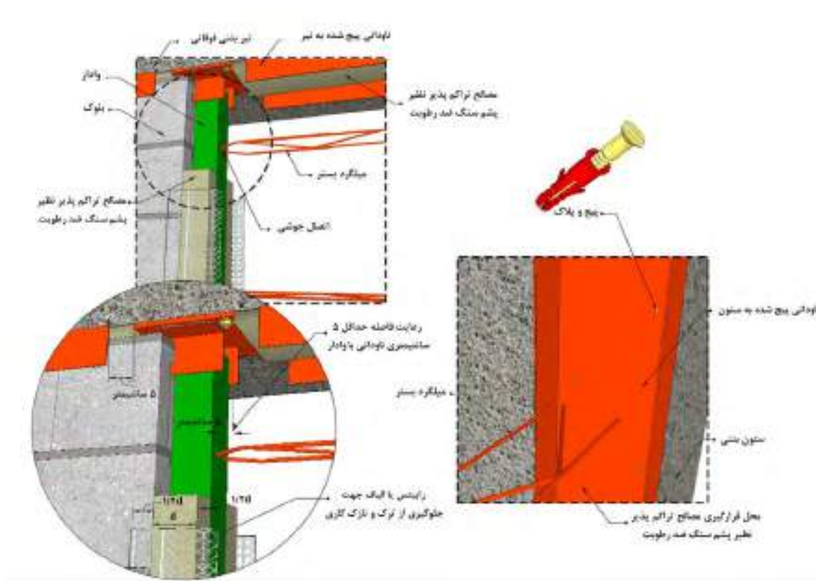
شکل ۱۱-۷- اجرای عایق پشم سنگ و مش الیاف یا رابیتس بر روی وادار
