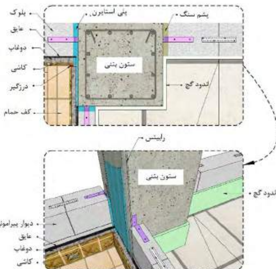
شکل ۱۱-۳- جزئیات اجرای کاشی بر روی ناحیه جداسازی شده بین دیوار و ستون در سرویس‌ها و آشپزخانه‌ها
