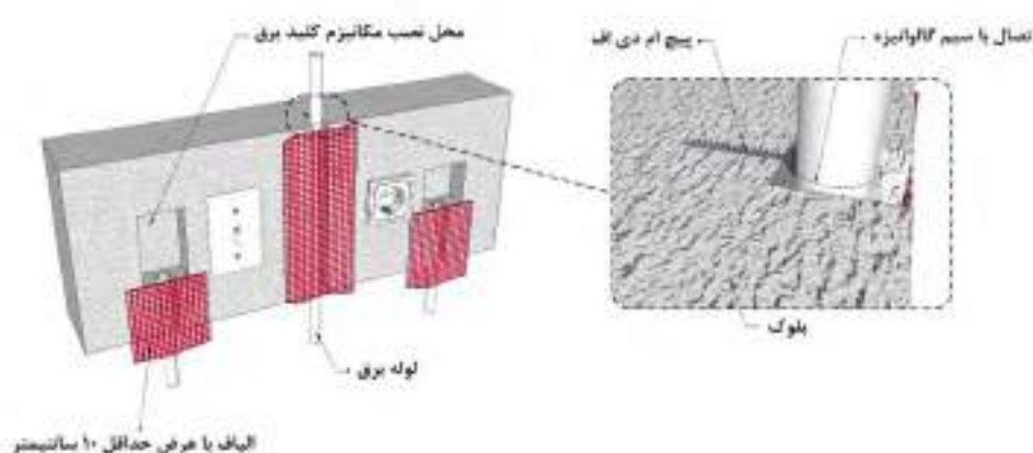
شکل ۹-۱۱- اجرای رابیتس یا مش الیاف بر روی شکاف های ایجاد شده در دیوار پیش از اجرای پوشش گچی جهت جلوگیری از ترک خوردگی اندود
