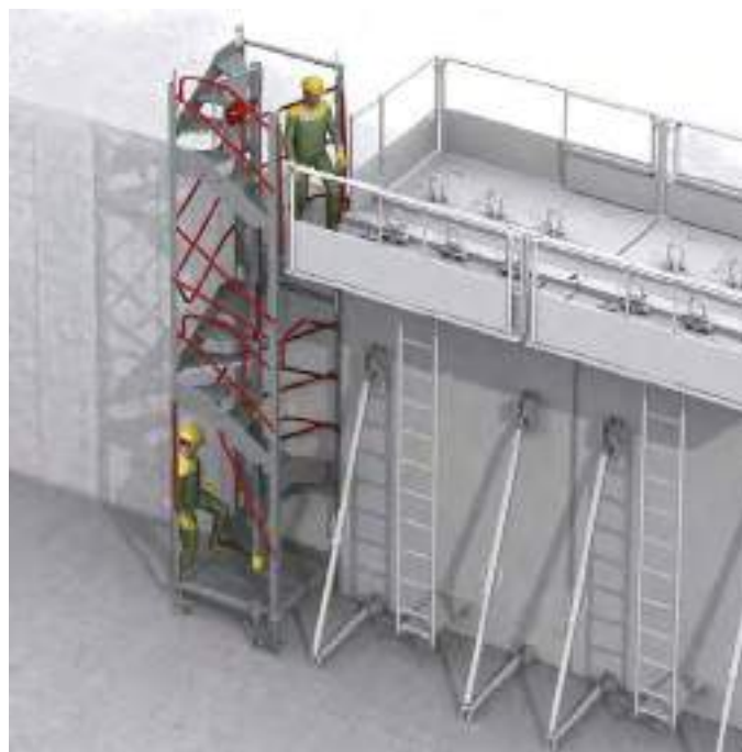
شکل ۵-۲۹- دسترسی ایمن به داخل گود
