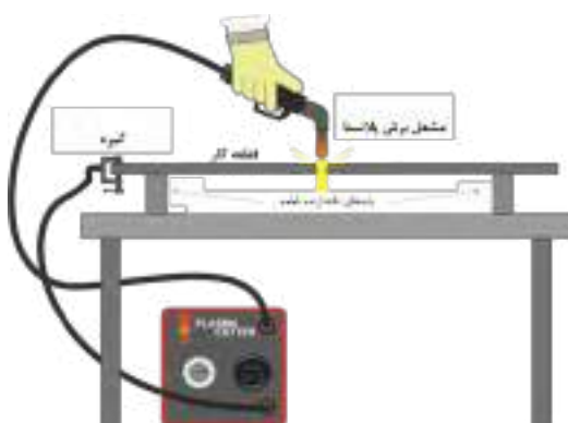
شکل ۴-۱۰- تصویر شماتیک برش با قوس پلاسما
