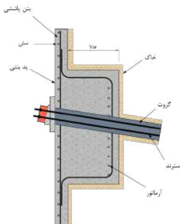
شکل ۵-۵- پد بتنی
