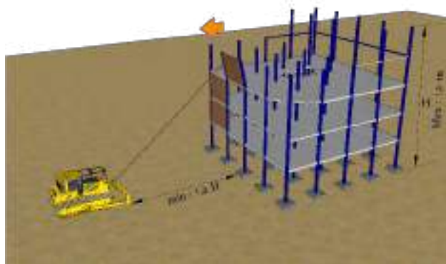
شکل ۴-۵- تخریب با کشیدن به وسیله طناب
