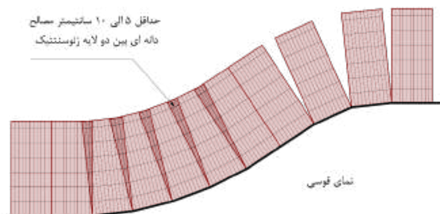
شکل ۵-۲۲- نمونه‌ای از نصب ژئوسنتتیک در دیوار با نمای قوسی
