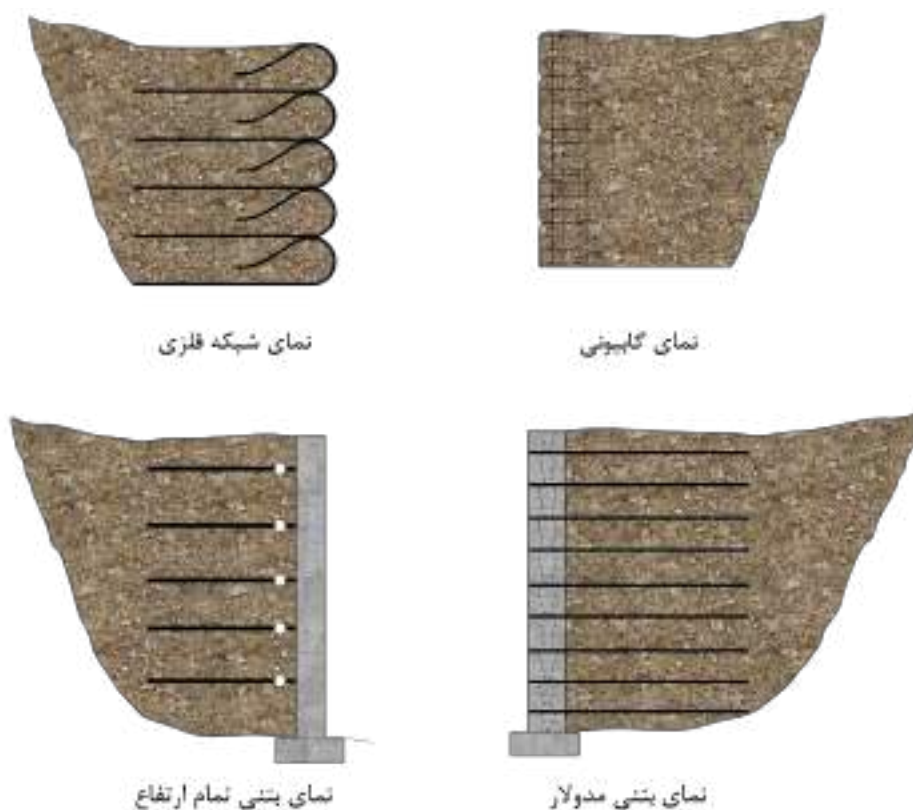
شکل ۵-۲۱- برخی از انواع نماهای معمول در دیوارهای خاک مسلح
