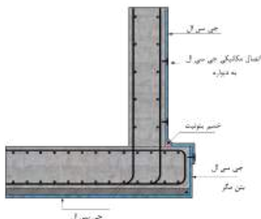
شکل ۵-۲۵- اجرای ژئوکمپوزیت رسی (جی سی ال) در اطراف پی
