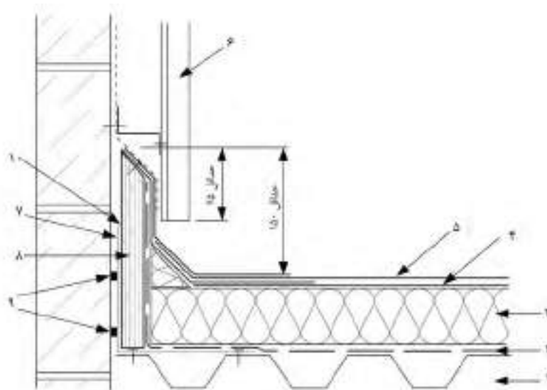
شکل ۱۰-۶- جان پناه- بام وارونه
