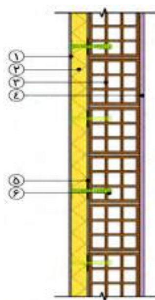
شکل ۱۰-۱۹- عایق کاری حرارتی با پلی استایرن و اندود نازک روی آن (ETICS)
