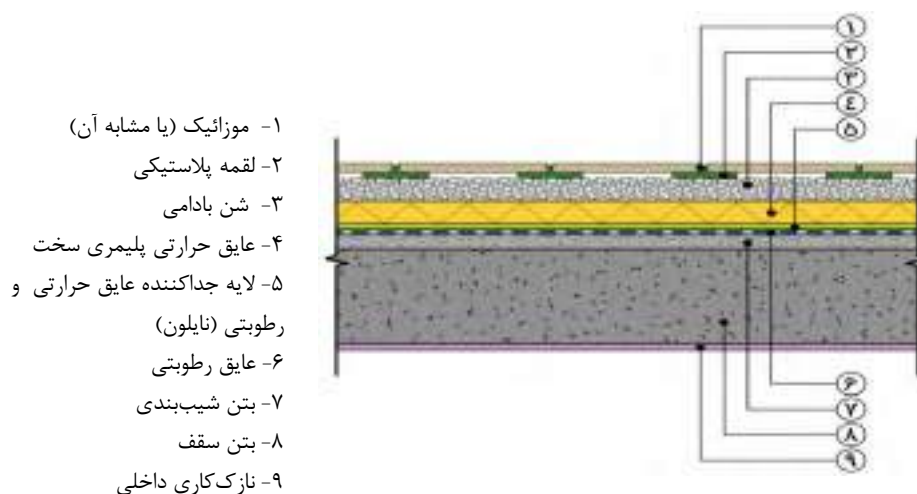
شکل ۱۰-۲۵- بام وارونه
