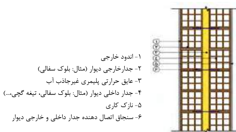
شکل ۱۰-۲۱- عایق‌کاری حرارتی دیوار به صورت میانی
