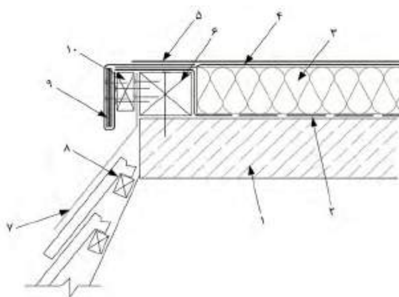
شکل ۱۰-۱۰-کناره بام
