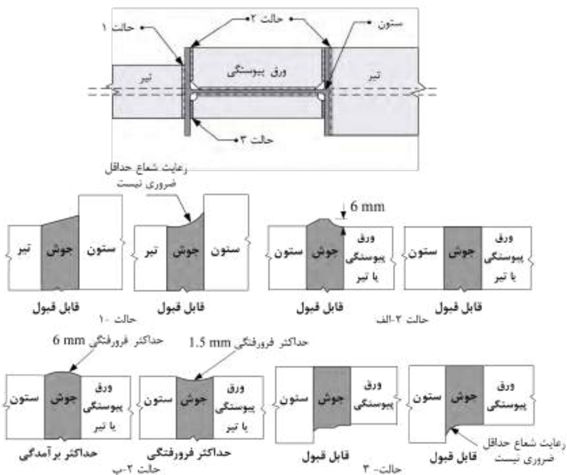
شکل ۷-۵- وضعیت‌های قابل قبول برداشتن ورق‌های گوشواره‌ای در انتهای جوش‌های شیاری با نفوذ کامل
