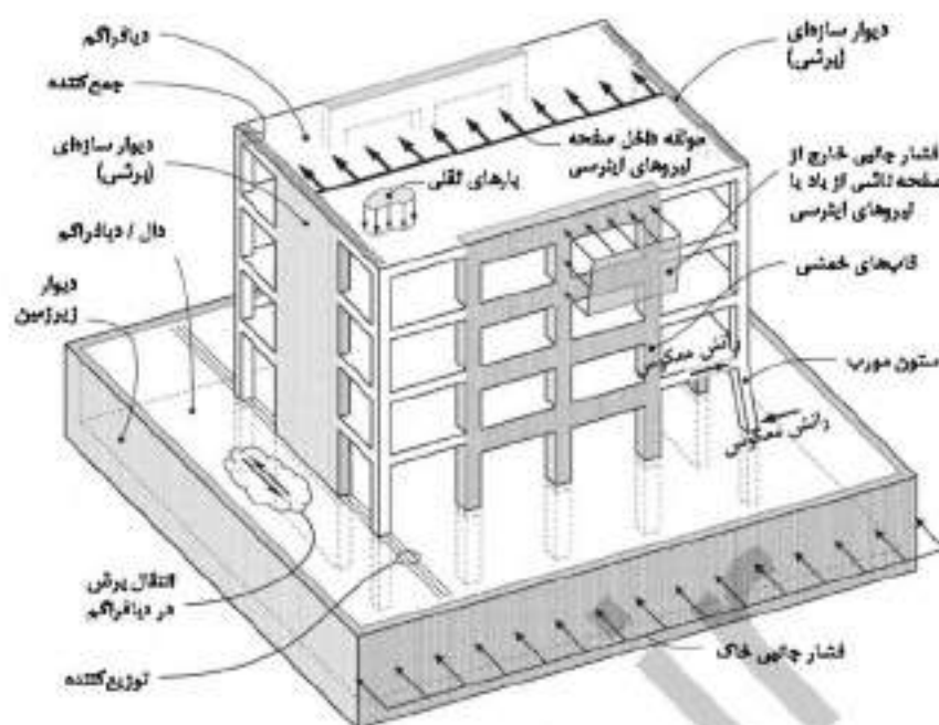
شکل ۹-۱۴-۱ نیروهای وارد بر دیافراگم
