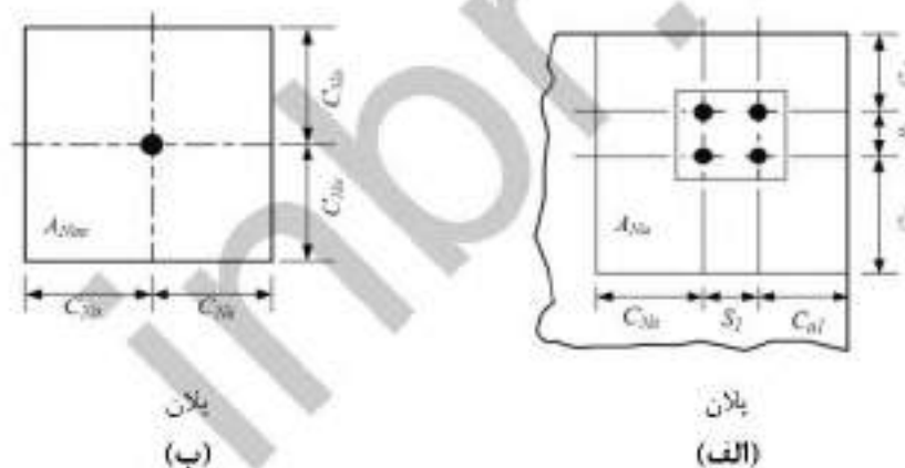
شکل ۵-۱۸-۹ روش محاسبه‌ی مساحت تصویر شده‌ی سطح گسیختگی، (الف) A_{No} (ب) A_{Nao}
