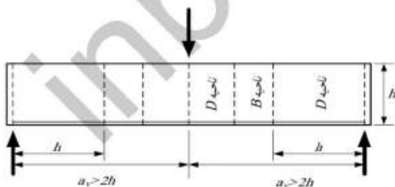
شکل ۹-ب-۳-۲ ناحیه‌های B و D در تیر با تکیه‌گاه ساده
