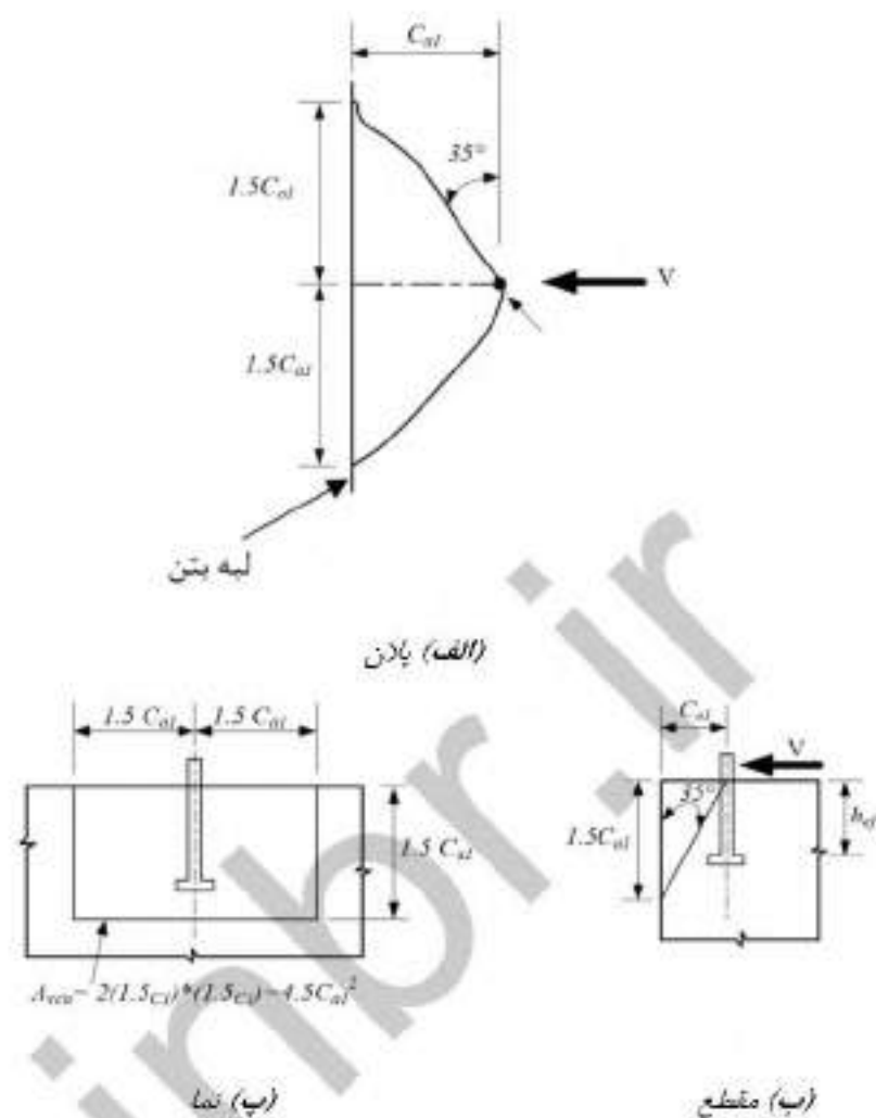
شکل ۹-۱۸-۶ مساحت تصویر شده‌ی سطح گسیختگی A_{req}
