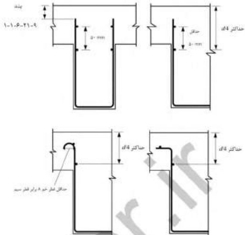
شکل ۲۱-۹ چهار در ناحیه فشاری خاموت L شکل متشکل از شبکه‌ی سیمی ساده‌ی جوشی شده
