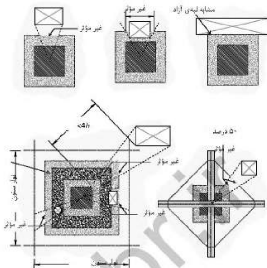
شکل ۹-۸-۱ تأثیر بارشو در دال بر سطح مؤثر مقطع بحرانی
