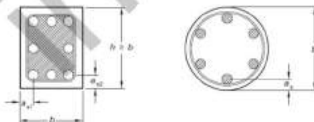
شکل ۹-۲-۱ فاصله‌ی محوری ( a ) در مقاطع اعضای سازه
