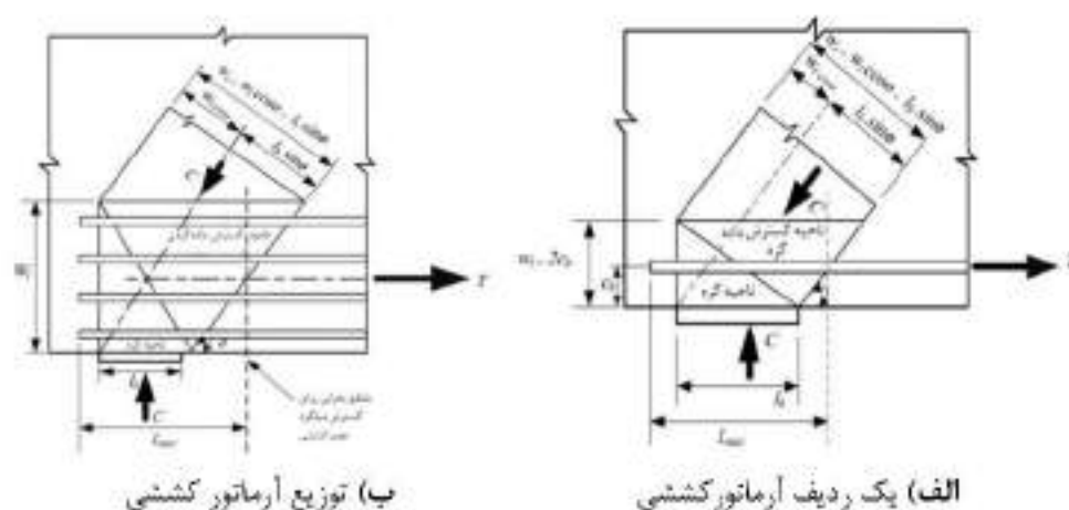
شکل ۹-۳-۲ نواحی بسط داده شده‌ی گره
