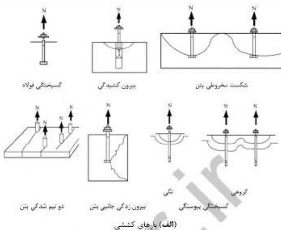
شکل ۱۸-۹-۲- انواع حالات تسمیه مهارها در کشش و برش
