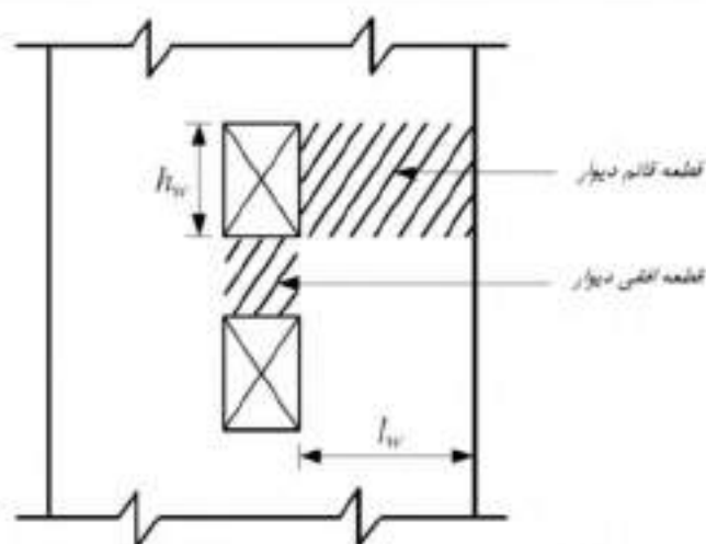
شکل ۹-۲۰-۱ دیوار سازه‌ای با بازشو
