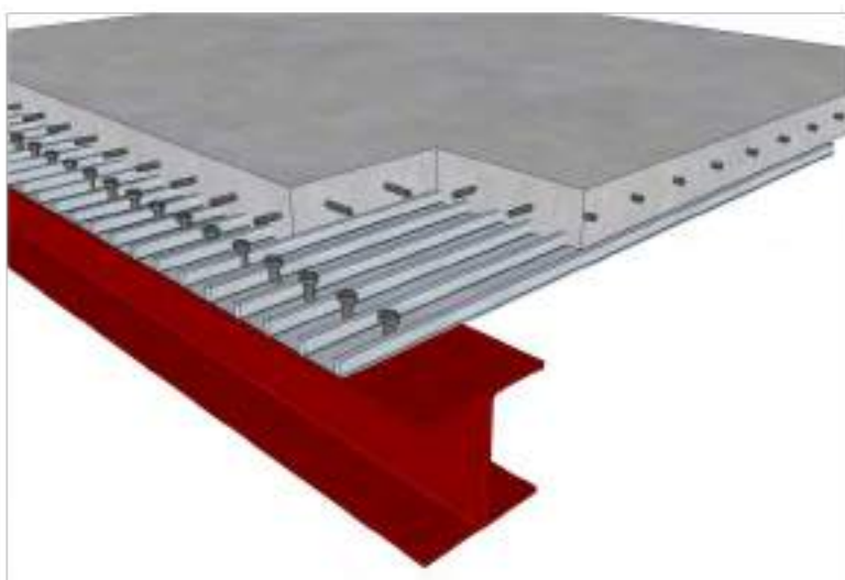
شکل ۶-۱۷- دال مرکب فولادی و بتنی
