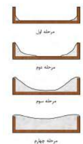
شکل ۶-۱۳- فرایند صحیح پاشش در گوشه‌ها
