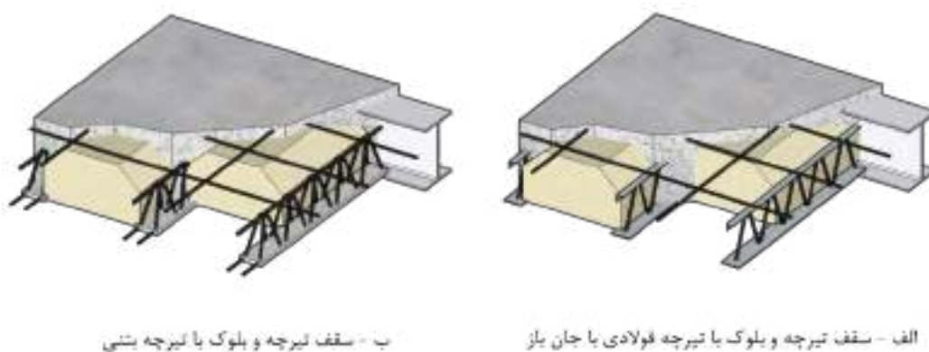
شکل ۶-۱۹ - شمای کلی از سقف تیرچه و بلوک
